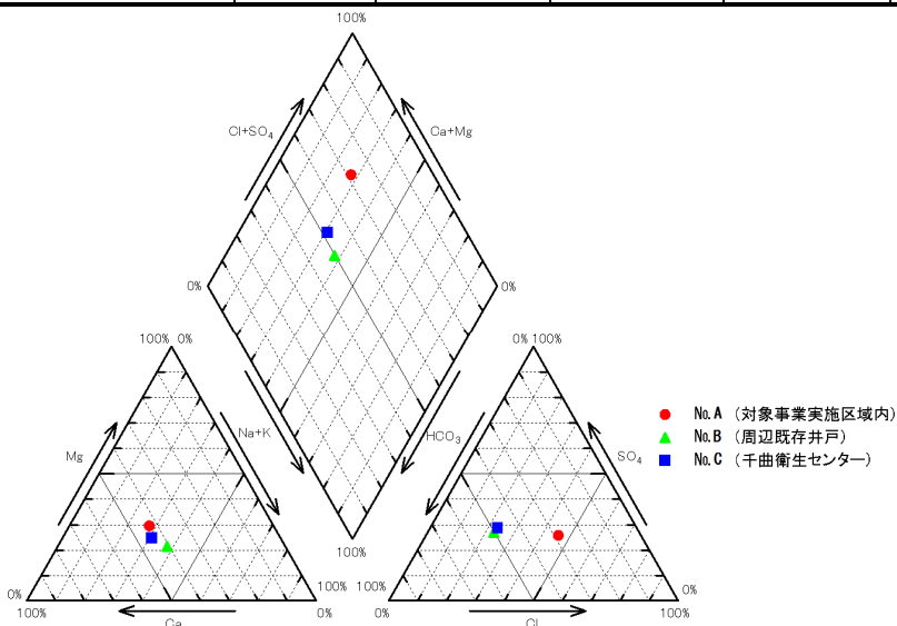
図 2 地下水質調査結果（トリリニアダイアグラム）
