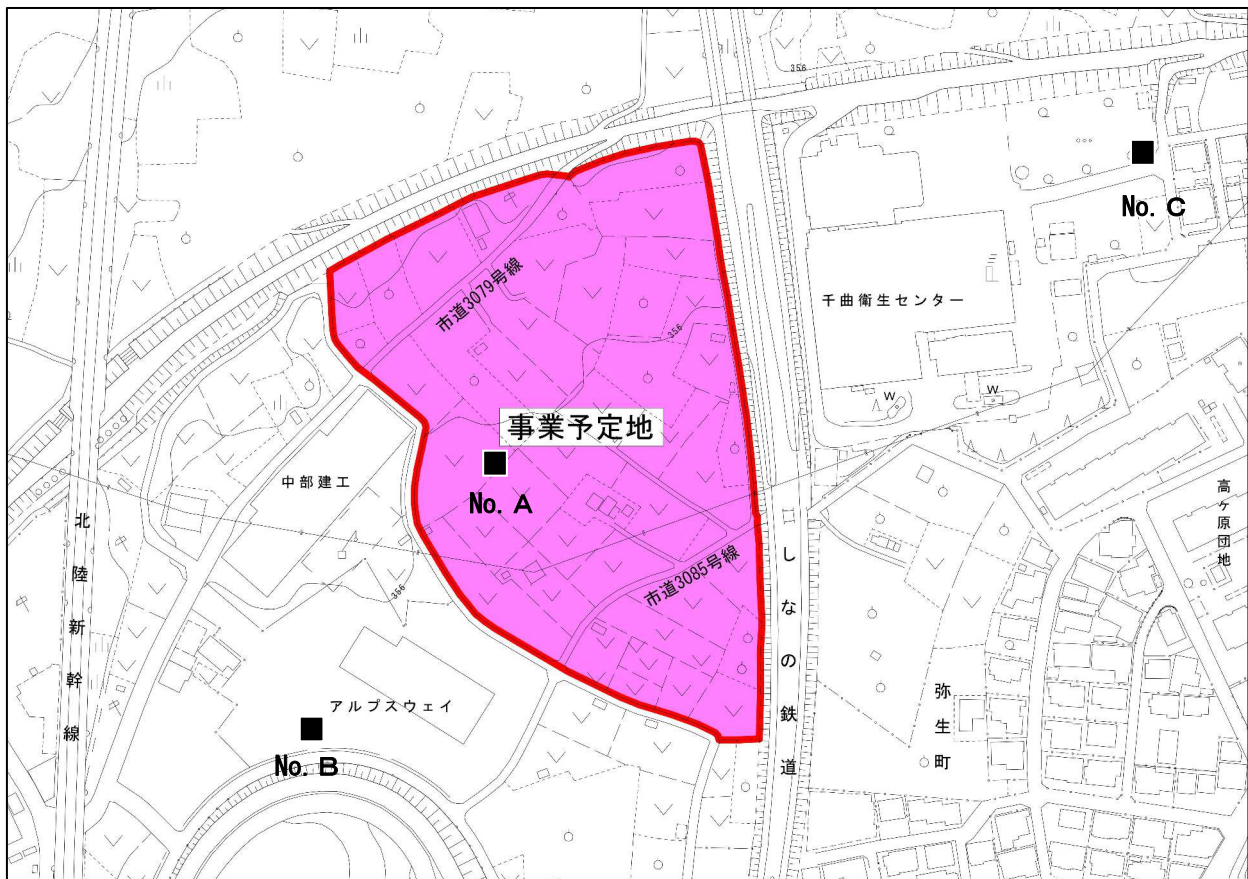
図 1 地下水質調査地点
