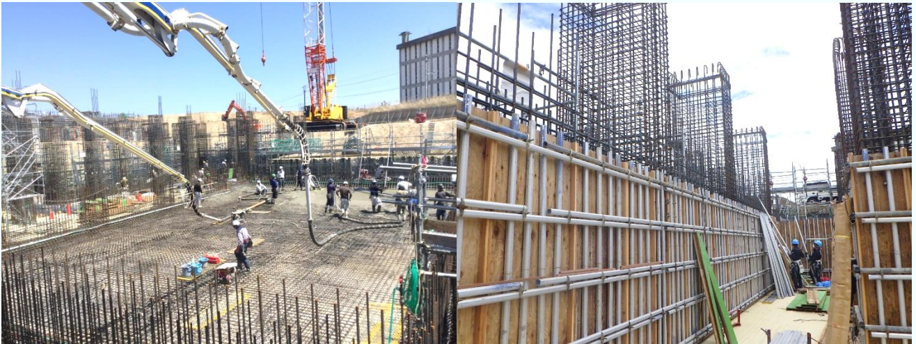
[ごみピットの底盤をつくっています]
