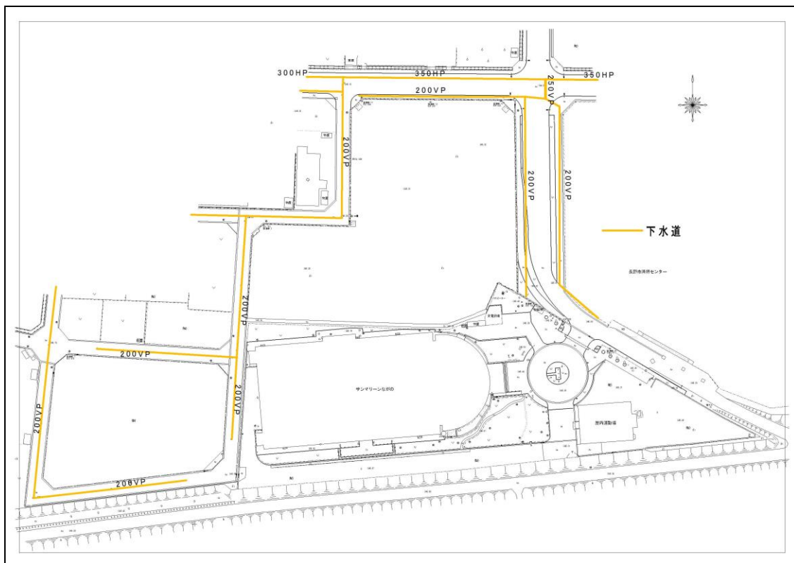
図 3 下水道の敷設状況
