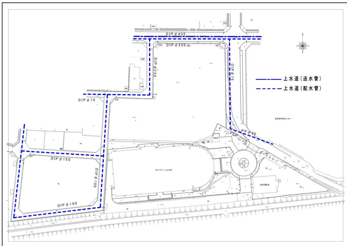
図 2 上水道の敷設状況
